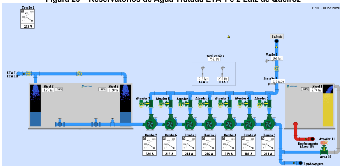
Figura 29 – Reservatórios de Água Tratada ETA 1 e 2 Luiz de Queiroz
