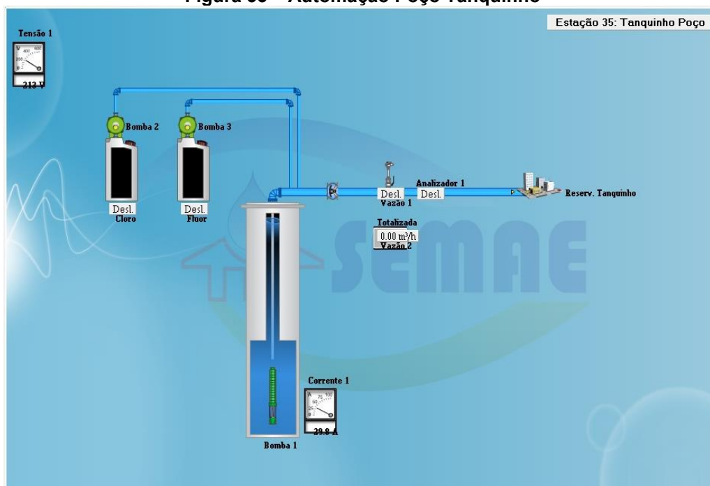
Figura 33 – Automação Poço Tanquinho
