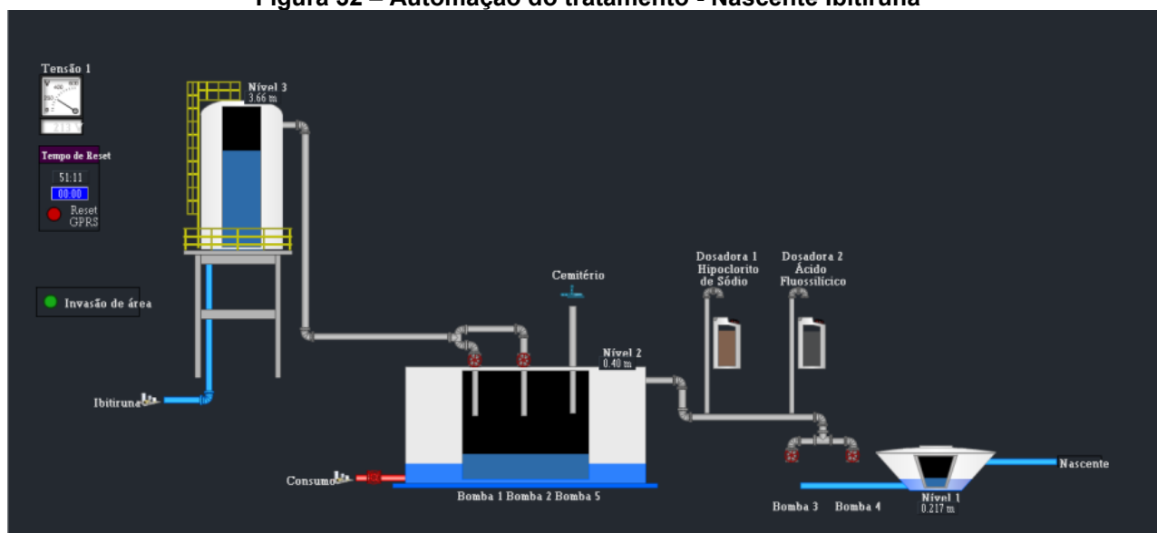
Figura 32 – Automação do tratamento - Nascente Ibitiruna
