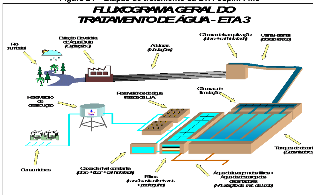
Figura 24 – Etapas de tratamento da ETA Capim Fino
