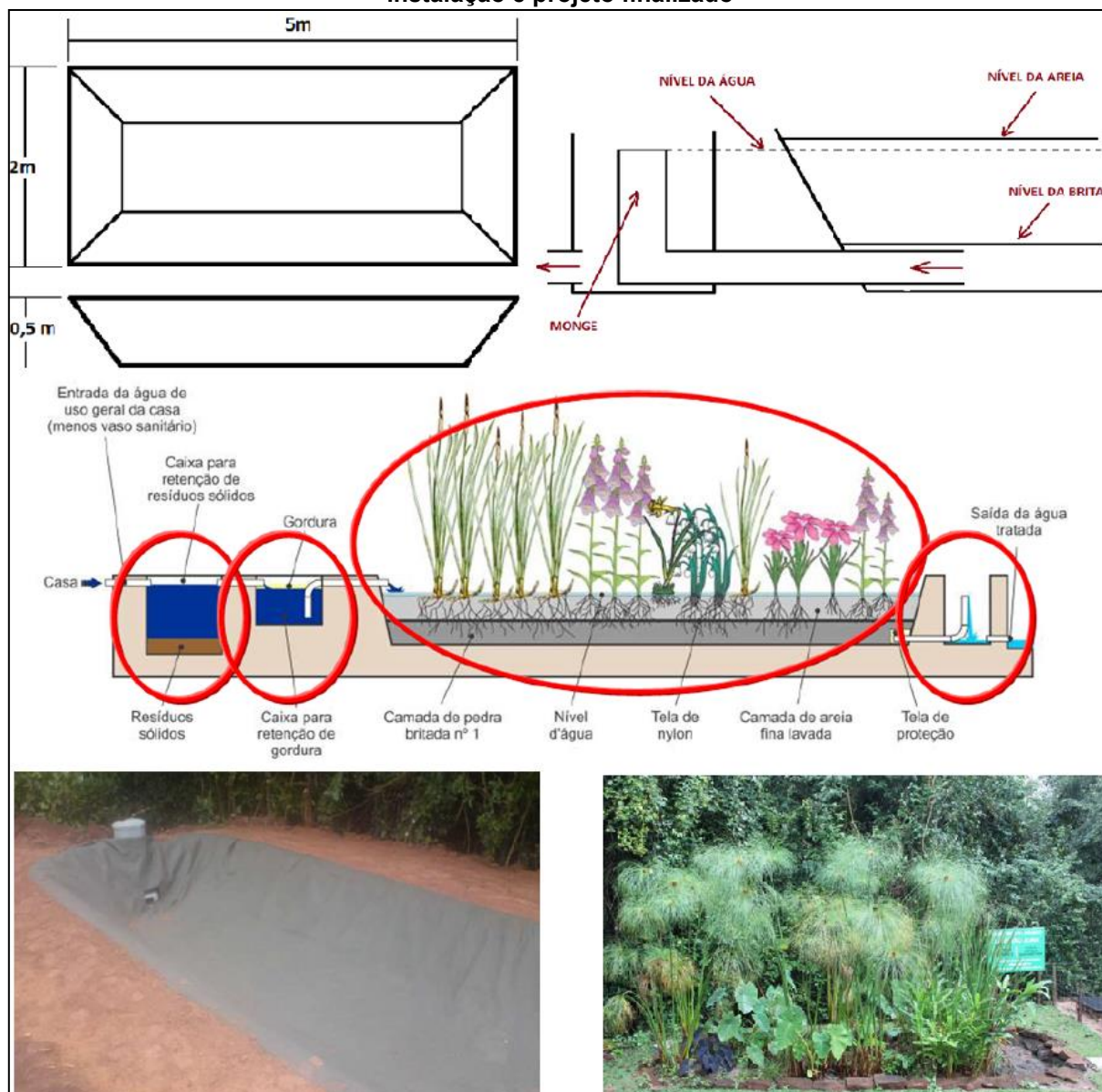
Figura 59 – Ilustração esquemática do Jardim Filtrante desenvolvido pela Embrapa e fotos reais da instalação e projeto finalizado
