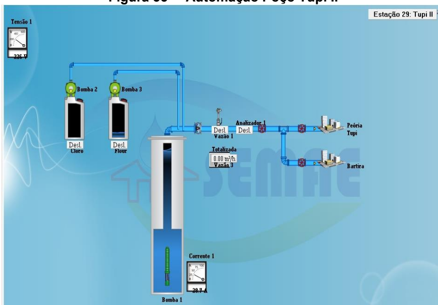
Figura 35 – Automação Poço Tupi II
