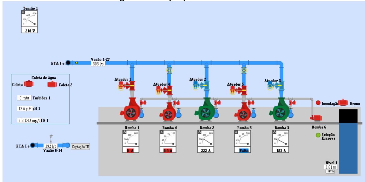
Figura 28 – Captação 1 rio Piracicaba
