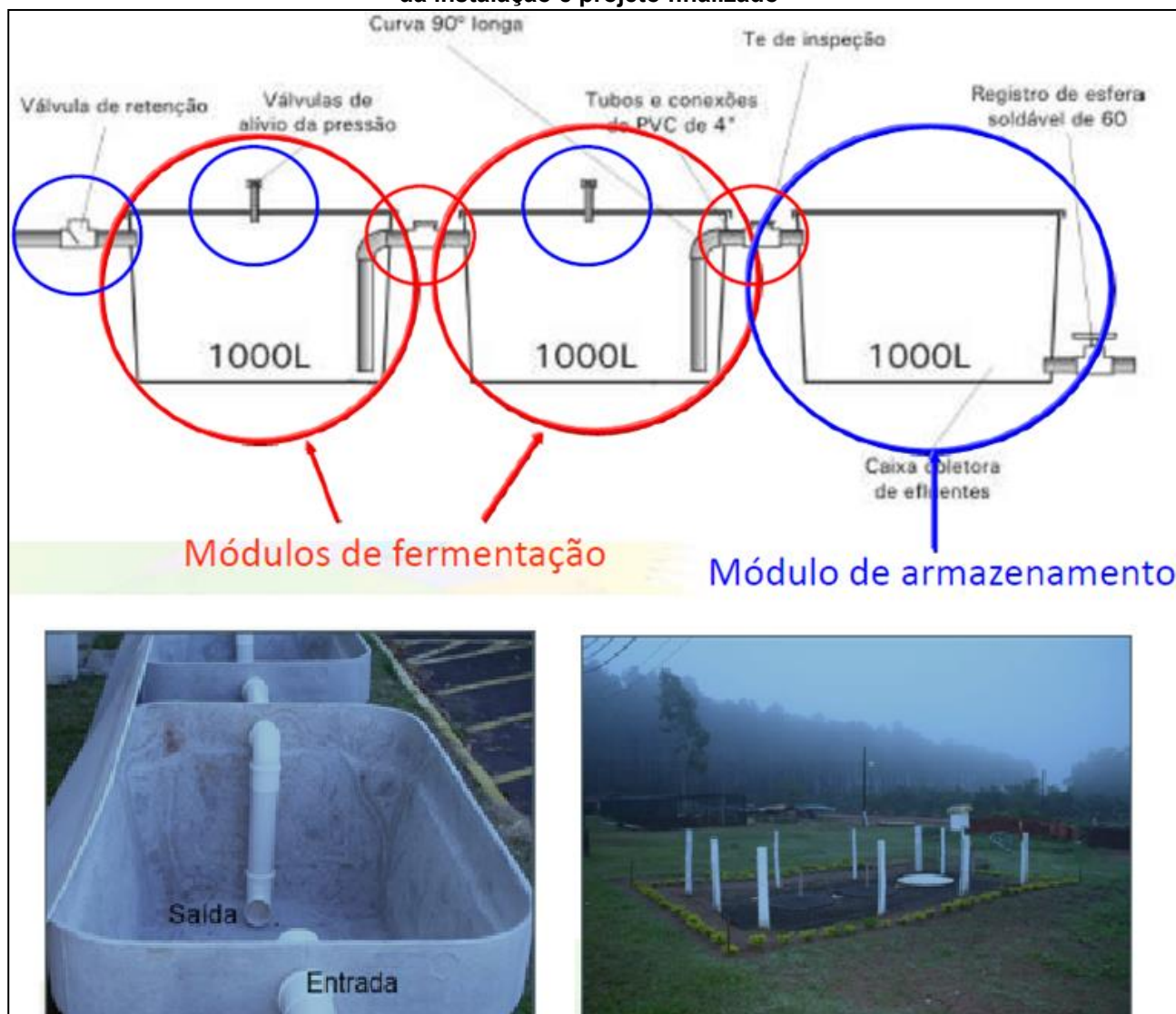
Figura 58 – Ilustração esquemática da fossa biodigestora desenvolvida pela Embrapa e fotos reais da instalação e projeto finalizado
