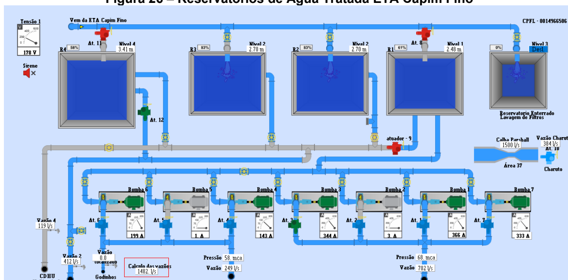
Figura 26 – Reservatórios de Água Tratada ETA Capim Fino
