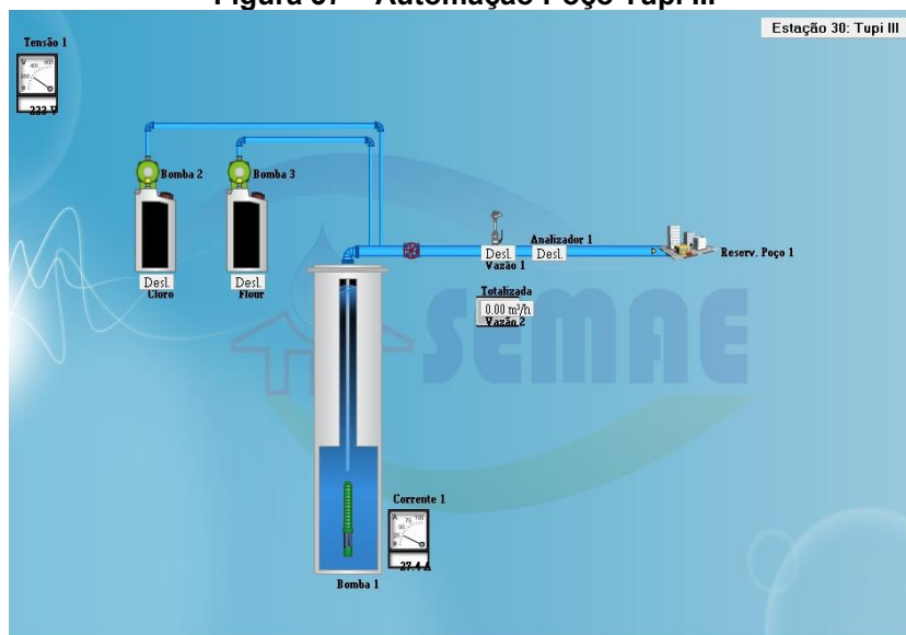
Figura 37 – Automação Poço Tupi III
