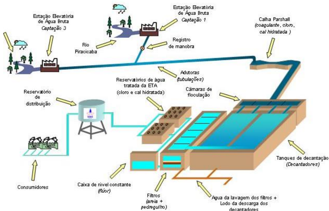
Figura 27 – Etapas de tratamento da ETA 1 Luiz de Queiroz (similar ETA 2)
