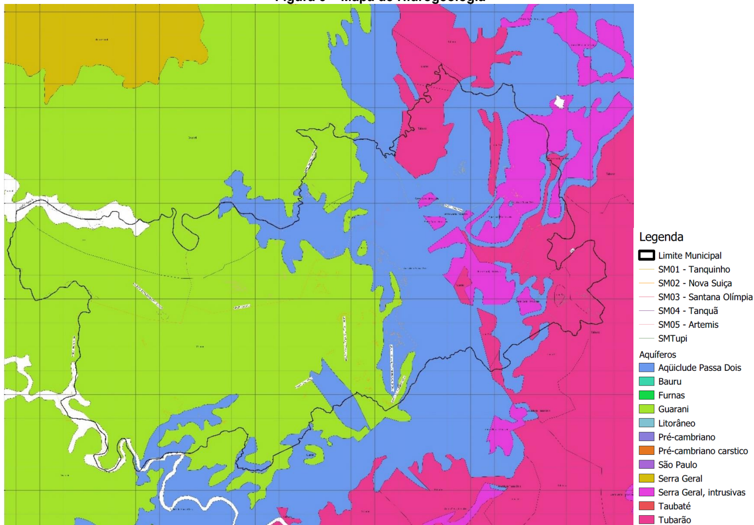
Figura 6 – Mapa de Hidrogeologia
