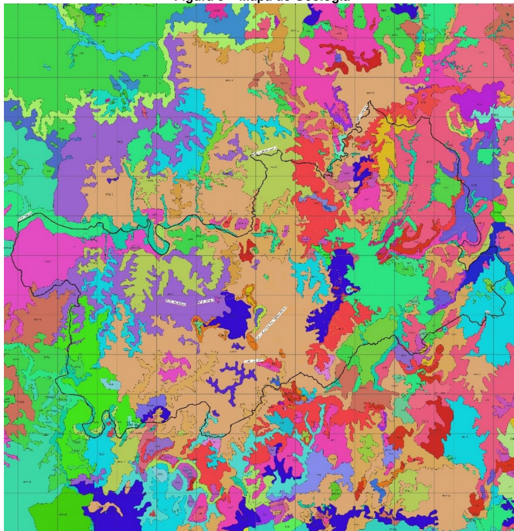
Figura 5 – Mapa de Geologia
