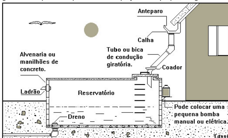
Figura 63 – Esquema simplificado de um projeto de captação de água de chuva.
