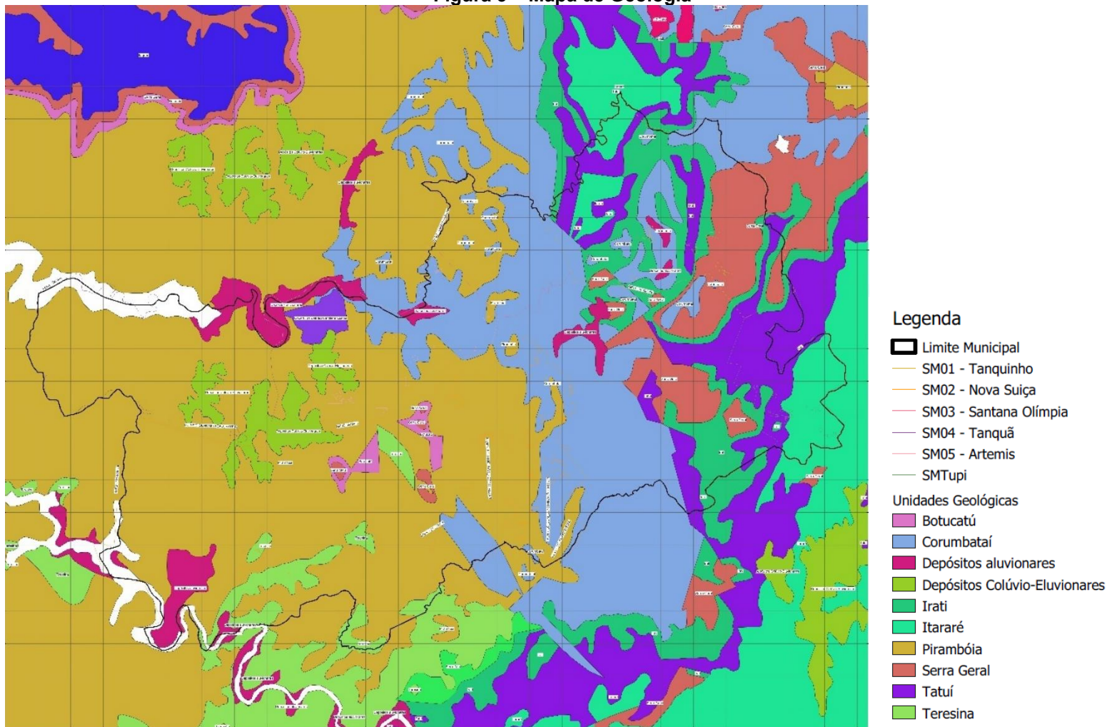
Figura 3 – Mapa de Geologia
