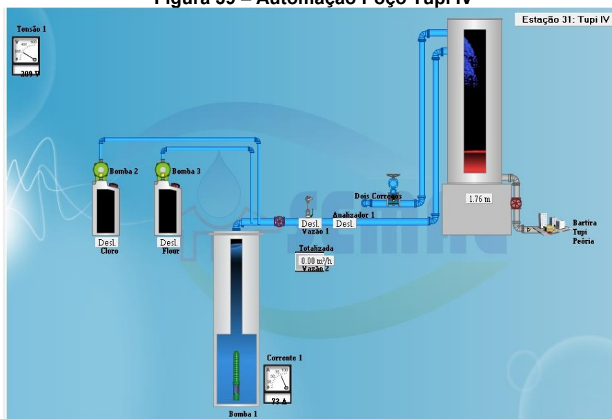
Figura 39 – Automação Poço Tupi IV
